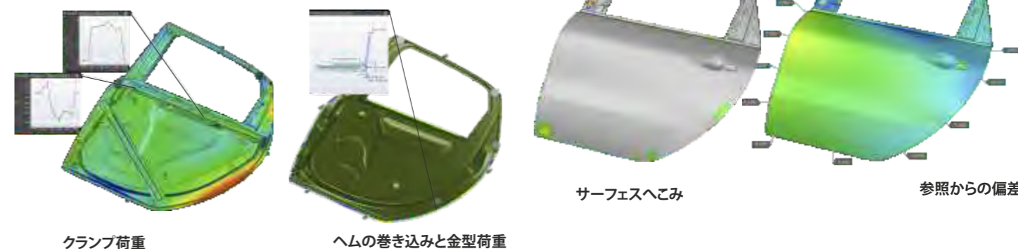
クランプ荷重 ヘムの巻き込みと金型荷重 サーフエスへこみ 参照からの偏差
